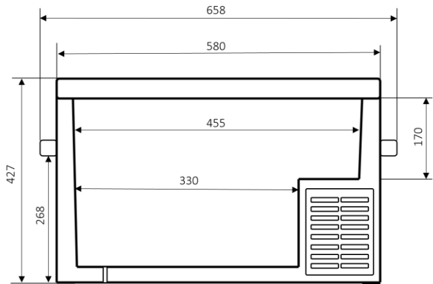
IceCube40
