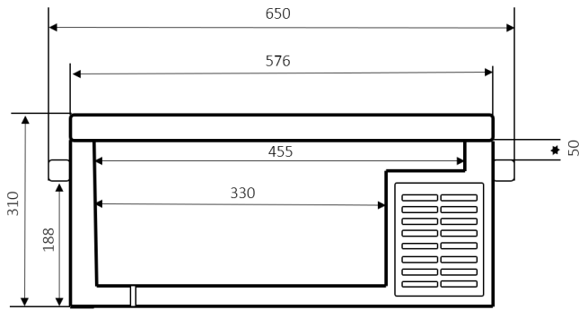
IceCube30
