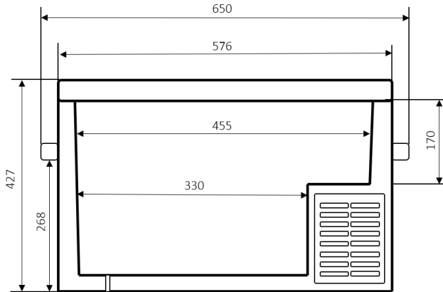
IceCube40
