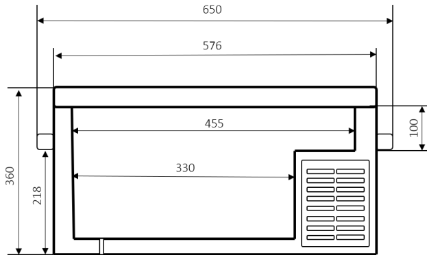
IceCube40
